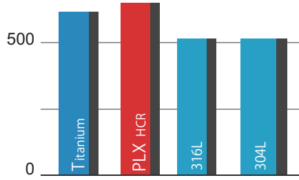
一般腐食 UIAA アンカー分類
